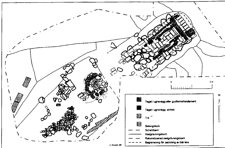
Fig. 5. Välbevarad senmedeltida klockgjutningsanläggning i Vendel. Det är mycket troligt att det var gjutare från ett av de undersökta Uppsalagjuterierna som utförde arbetet i Vendel. En klockgjutning är ett exempel på metallhantering med högt prestigevärde och symboliska förtecken. Bild: J. Anund.
