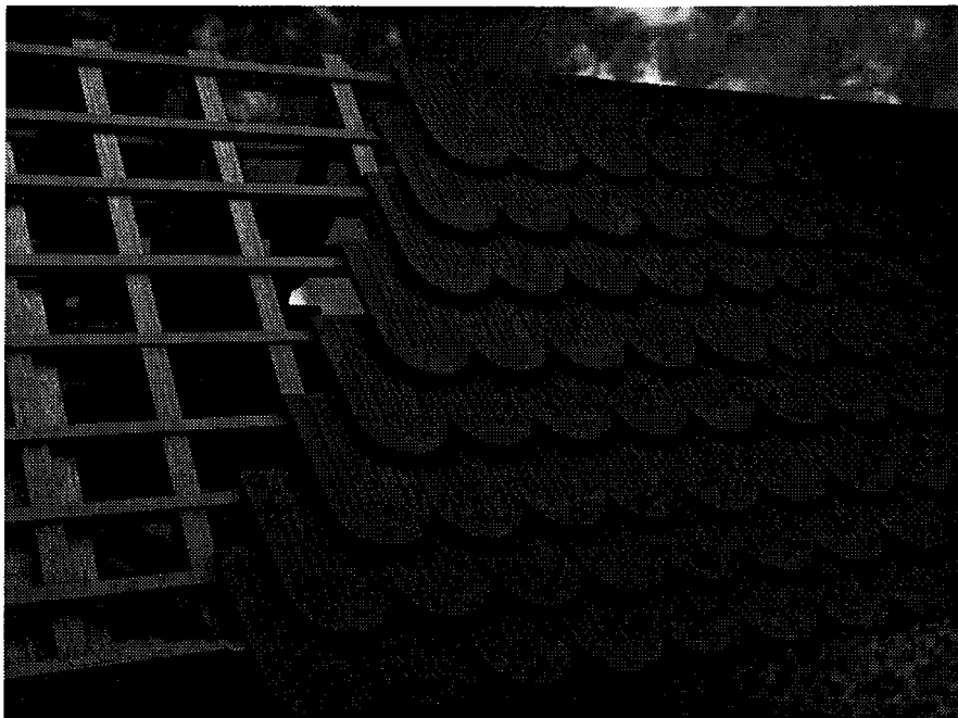
Figur 4. På grundval av utgrävningsresultaten förefaller det som om plattformade taktegel varit i bruk under en relativt ganska lång period, kanske allt ifrån medeltiden ända till branden i början på 1700-talet (3D-datamodell).
