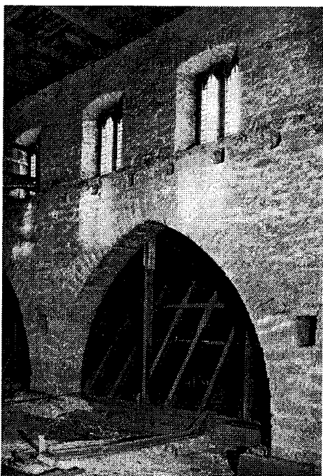
Fig. 10. Klerestorieetagen eller magasinsloftet ved Mariakirken i Visby. Foto 1975 i SvK 175, 1978.
